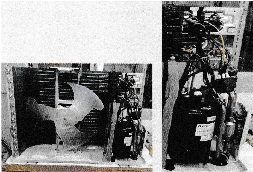
Photos des composants de l'unité extérieure
